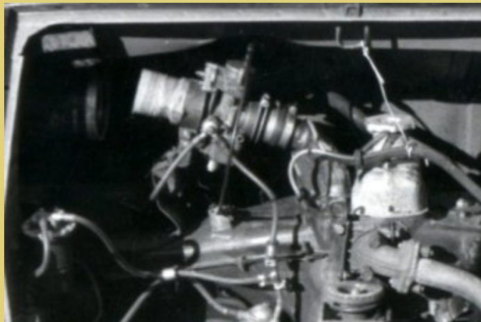
Jedno z udoskonaleń A. Szyjkowskiego: Fiat 126p z gaźnikiem Dellorto od motoru żużlowego. Obok: początki w garażu babci (1978) [1]
